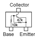
2SC4047 (ZY) (Lot.1) (Q1702)
