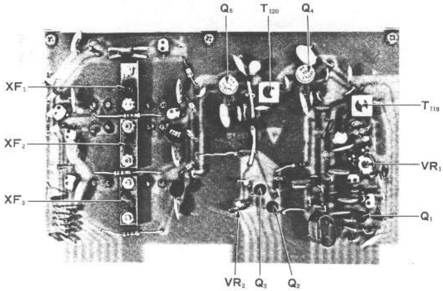
Fig. 15 IF UNIT
